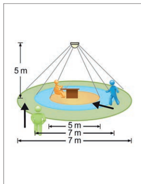
Sensor armatuur-opbouwset
